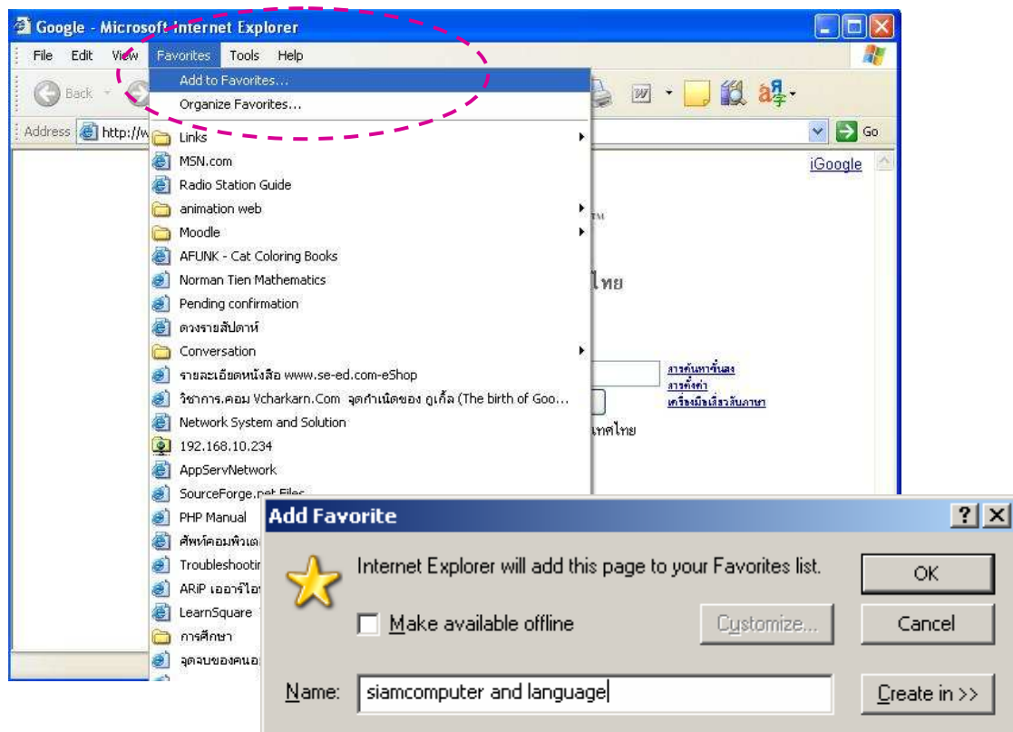
ภาพที่ 3-1 แสดงขั้นตอนการเก็บเว็บไซต์ที่ชื่นชอบ (Favorites)
